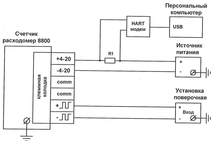
Рисунок А.1 – Схема подключения расходомера при определении погрешностей измерения объема или объемного расхода с использованием программы программ AMS или Prolink
