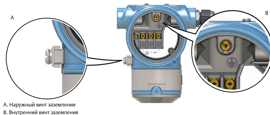
Рисунок 4-3. Винты заземления
