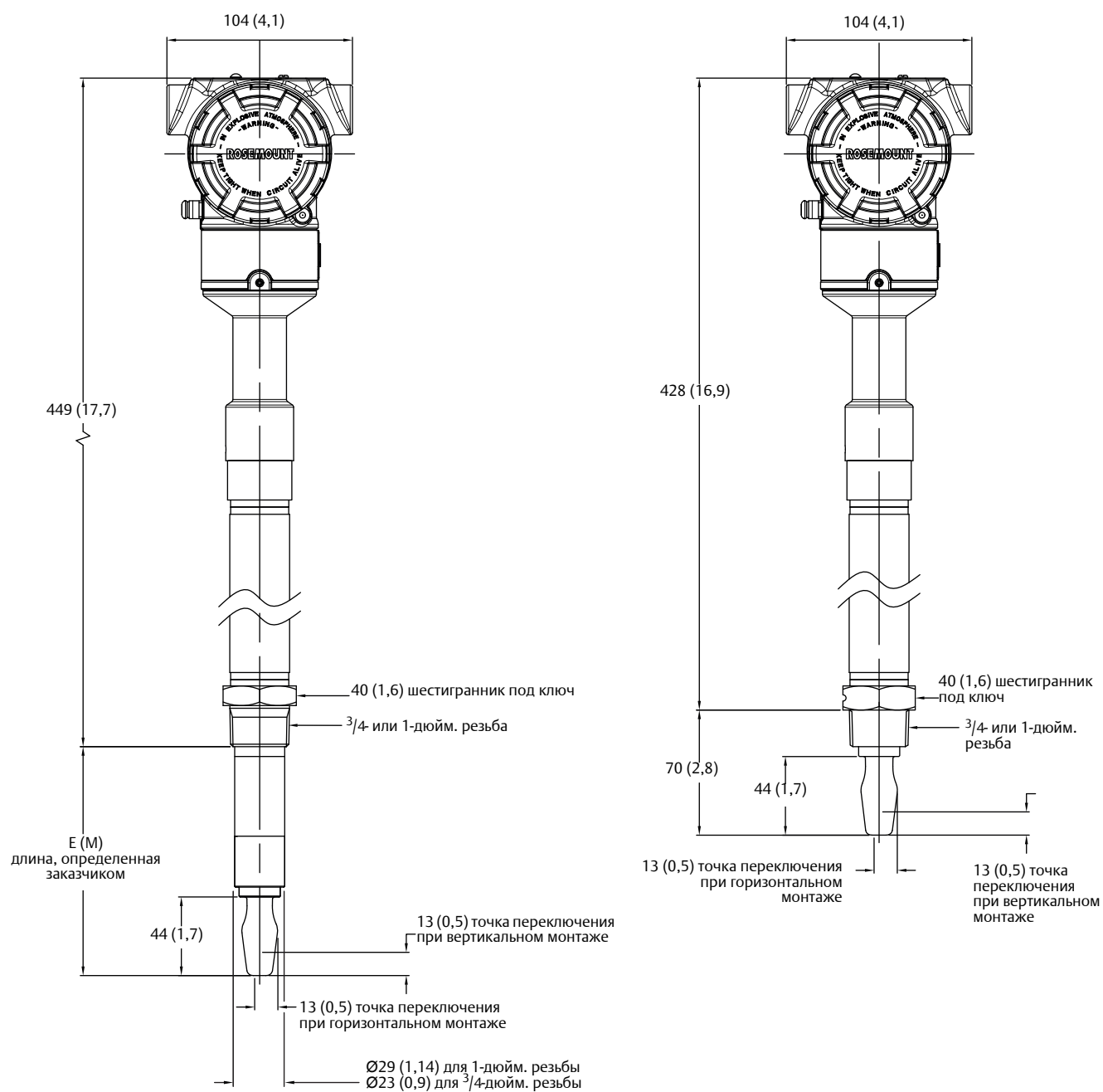
Рисунок А-5. \frac{3}{4} - и 1-дюйм. резьбовое технологическое соединение (диапазон высокой температуры, вилки всех вариантов длины)
