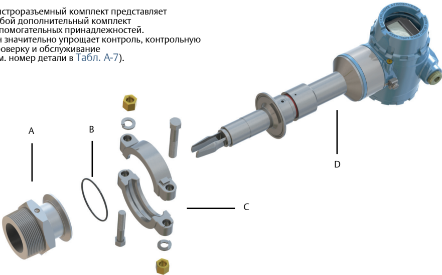
Рисунок А-12. Быстроразъемный комплект.
