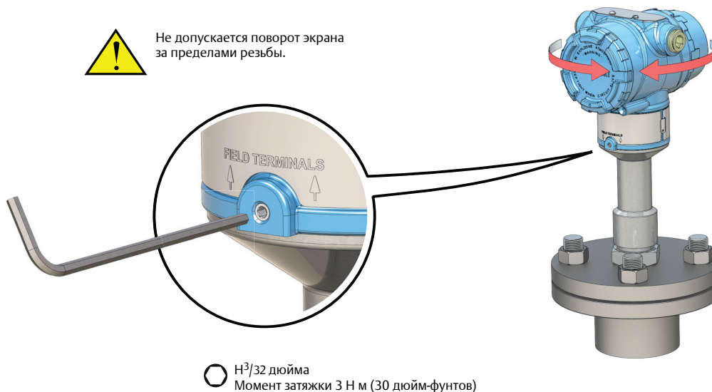
Рисунок 3-4. Поворот корпуса
