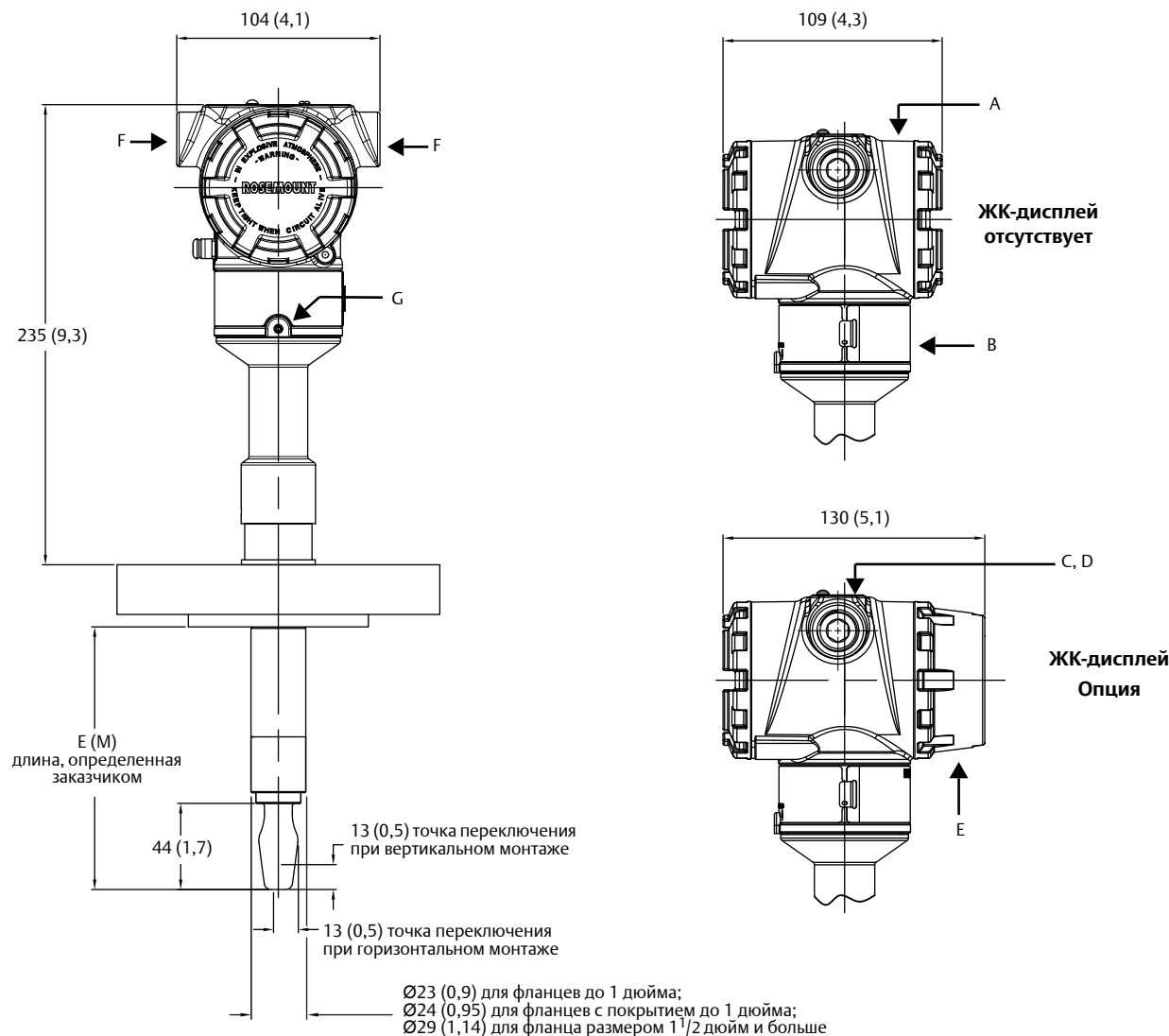
Рисунок А-10. Фланцевое технологическое соединение (средний диапазон температуры, удлиненная вилка)
