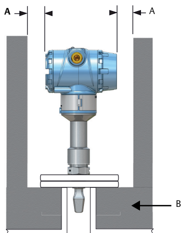
Рисунок 3-16. Изоляция
