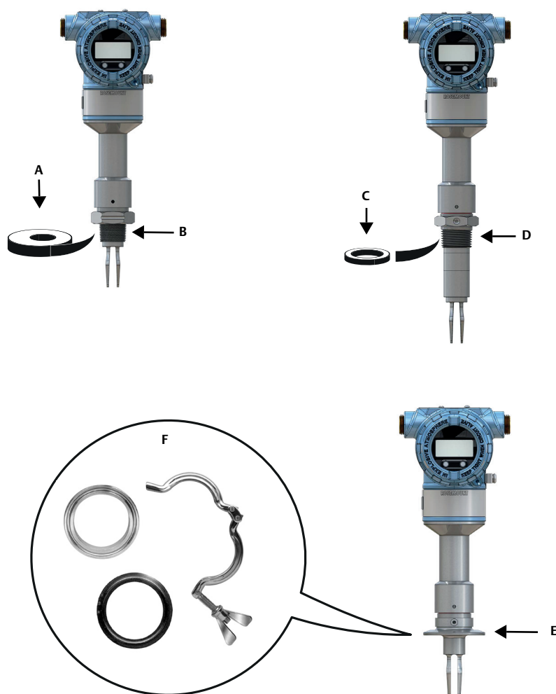
Рисунок 3-11. Изоляция технологического соединения
