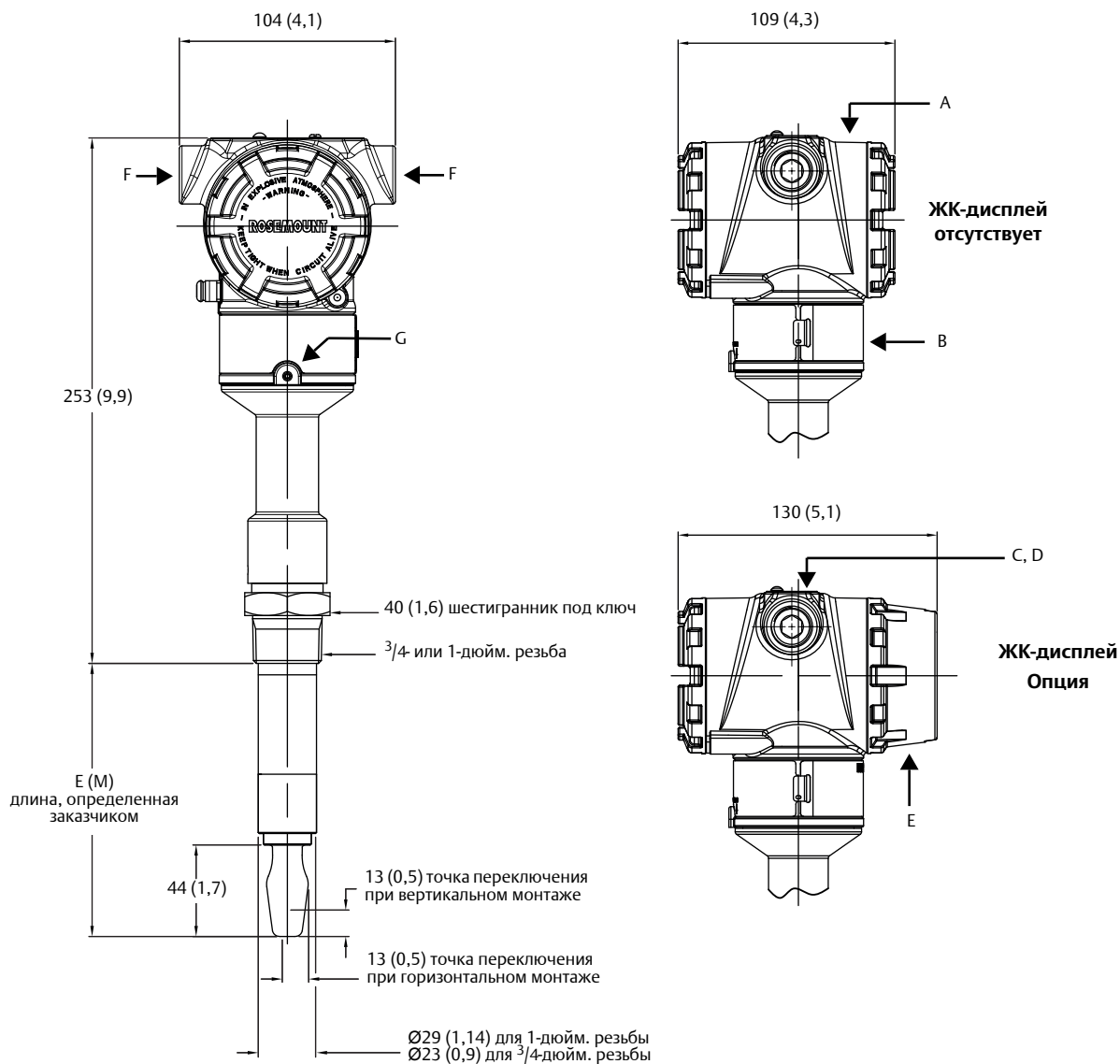
Рисунок А-4. \frac{3}{4} - и 1-дюйм. резьбовое технологическое соединение (средний диапазон температуры, удлиненная вилка)
