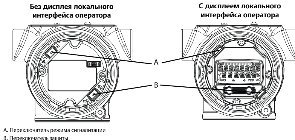
Рис. 2-6. Переключатель защиты и реле сигнализации
